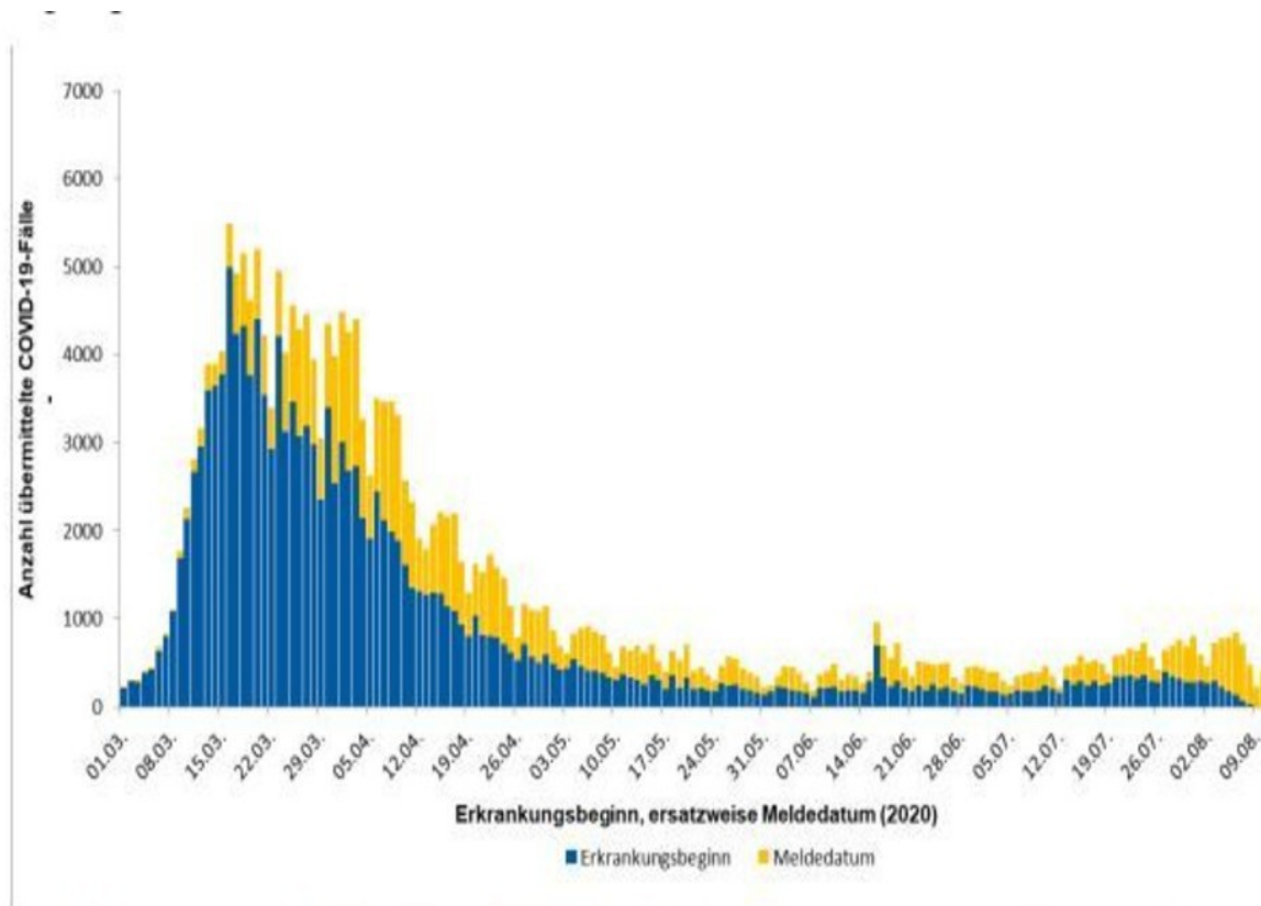
Abbildung 3: Anzahl der an das RKI übermittelten COVID-19-Fälle nach Erkrankungsbeginn, ersatzweise nach Meldedatum. Dargestellt werden nur Fälle mit Erkrankungsbeginn oder Meldedatum seit dem 01.03.2020 (11.08.2020, 0:00 Uhr).
